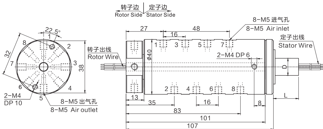
3008004 (8进8出, 4~6mm气管) +6~36路信号系列尺寸图 (适用于电磁阀与感应开关)
