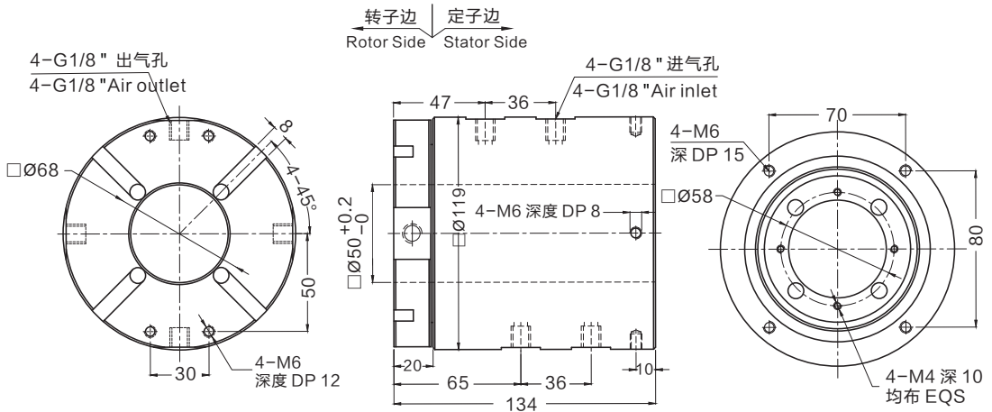
3504006 (4进4出, 6~8mm气管, 孔径50mm, 纯气动旋转接头) 尺寸图
