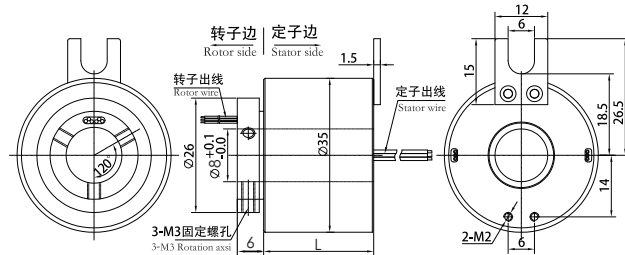
2路、3路、4路、6路规格图纸
