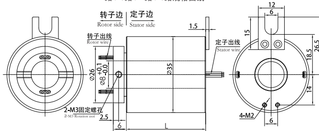
8路、10路、12路规格图纸
